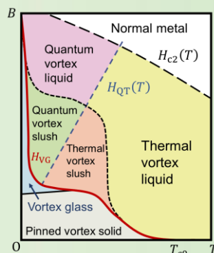
Bi系高温超伝導体の 磁場-温度相図
