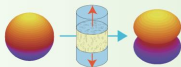
異方的媒質中での 3 Heポラー超流動
