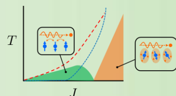
Doniach 相図
