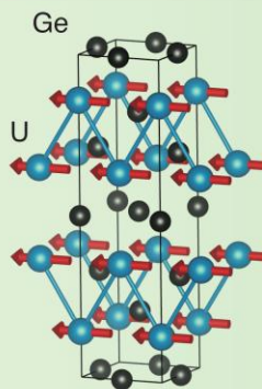
超伝導体 \text{UGe}_2 の 結晶・磁気構造
